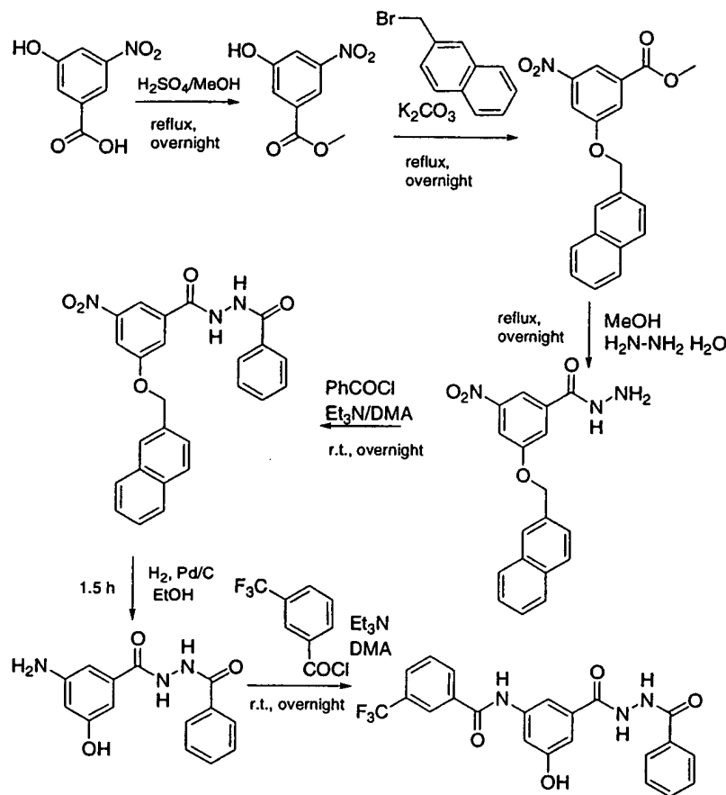
Scheme VI
